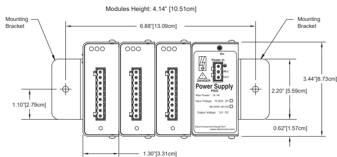
Nexus® I/O Modules Front View
